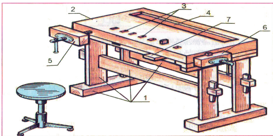
Мизи дуредгарӣ: 1 - асос; 2 - сарпӯш; 3 - сӯрохиҳо барои фона; 4 - нова; 5 - гирои пеш; 6 - гирои қафо; 7 - ангуштҳои ҳаракатнок.
