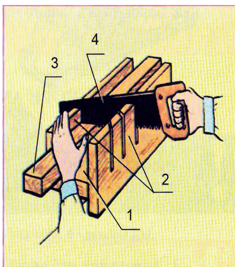
Арракунӣ бо ёрии стуло: 1- асос; 2 - девораҳо; 3 - тахтама- солах, 4 - арра.
