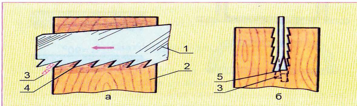
Расми 25. Буриши барқад: а - намуд аз паҳлу, б - намуди буриши арра; 1 - арра, 2 - масолеҳ, 3 - аррамайдаҳо, 4 - нӯги дандона, 5 - тегаи бурандаи дандона.
