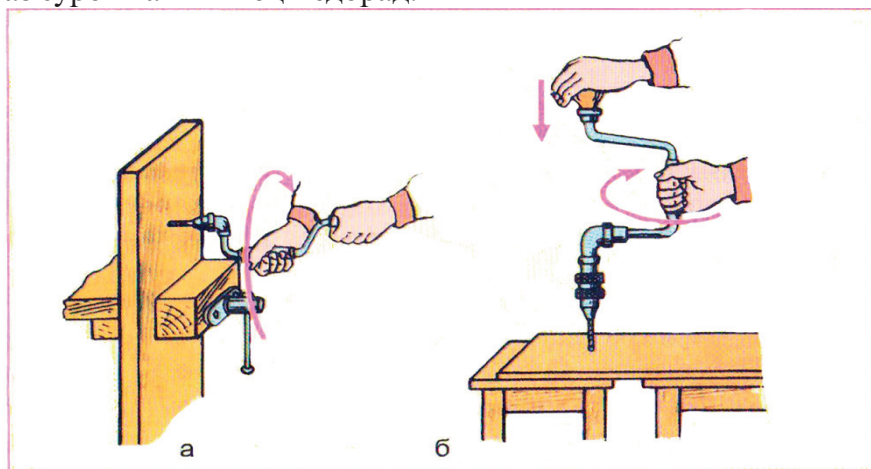
Расми 35. Тарзҳои пармакунӣ: а - дар гирои мизи дуредгарӣ; б - дар рӯйи сатҳ.
