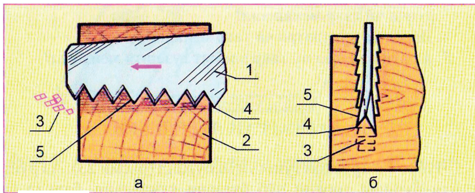
Расми 24. Буриши кӯндаланг: а - намуд аз паҳлуи арра; б - намуд аз буриши: 1 - арра; 2 - масолеҳ; 3 - аррамайда; 4 - нӯги дандонаи арра; 5 - тегаи бурандаи дандонаи арра.
