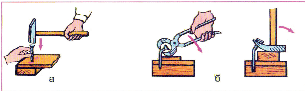
Мехкӯбӣ (а) ва мехкашӣ (б).
