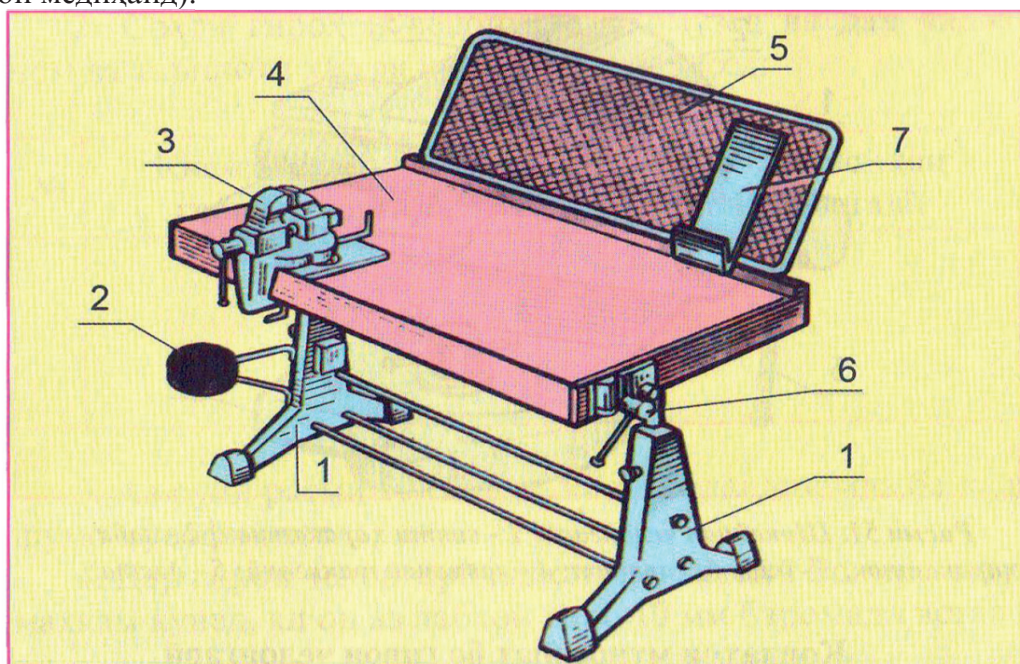
Расми 49. Мизи челонгариӣ универсалӣ: 1 - асос; 2 - ҷойи нишааст; 3 - шиканҷаи челонгарӣ; 4 - сарпӯш; 5 - симтӯри муҳофизатӣ; 6 - гирои миз; 7 - ҷойи гузоштани ҳуҷҷатҳои техникӣ.
