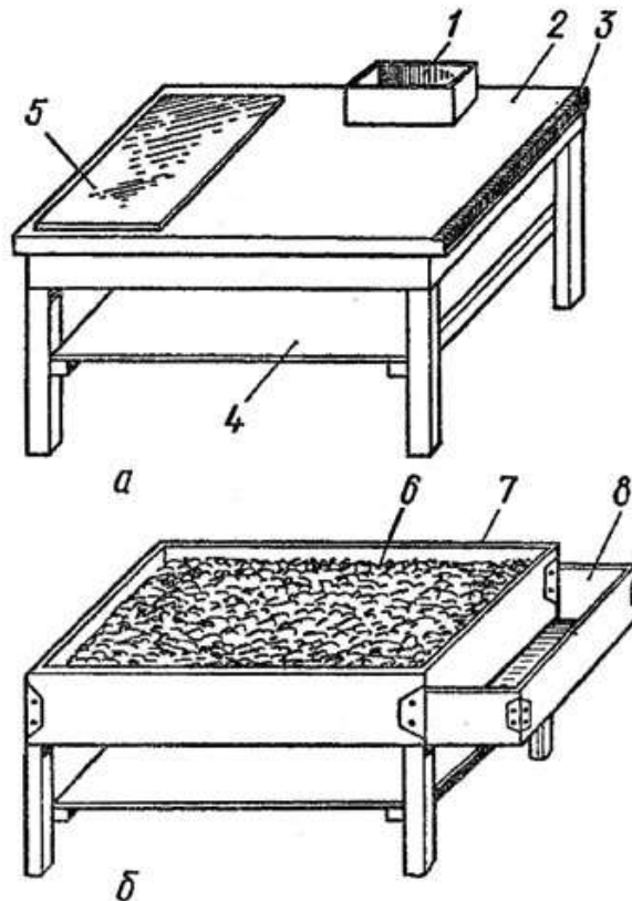
Расми 4. Чои кори сикказан: а) мизи корӣ, б) қуттӣ бо қум: 1. қуттӣ барои асбобҳо; 2. рӯи миз; 3. қунҷаки пӯлодӣ; 4. раф барои халта бо қум; 5. лавҳаи пӯлодӣ; 6. қум; 7. тарафҳои қуттӣ; 8. чой барои асбобҳо.
