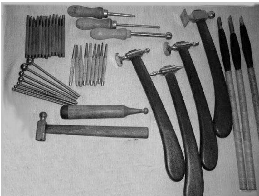
Расми 3. Намунаи асбобҳо барои сикказанӣ
