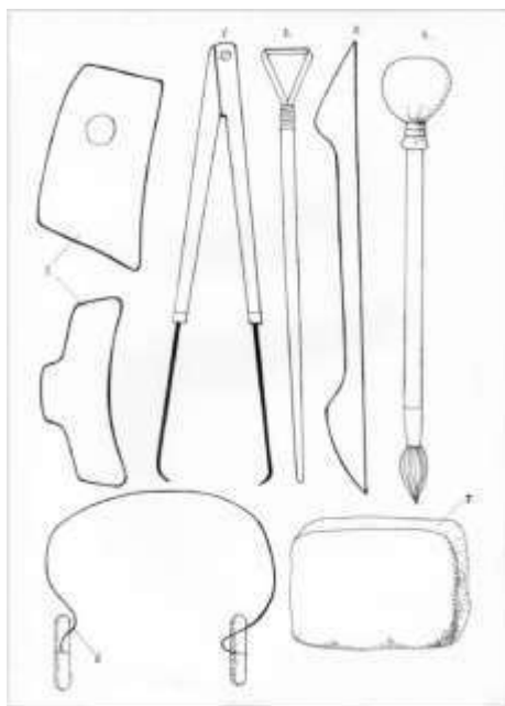
Асбобҳои асосии кулолгарӣ: 1 – паргори гафсиченкунанда, 2 – ҳалқа, 3 – халачӯб, 4 – мӯйқалам бо обчинак (губка), 5 – қолабҳо, 6 – сим, 7 – обчинак (губка)
