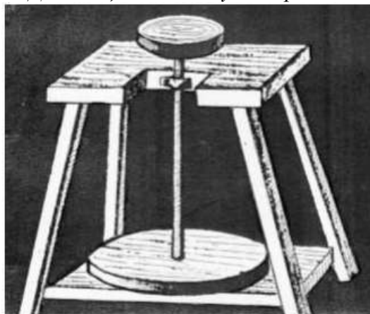
Дастгоҳи кулолгарии бо пой ҳаракатдиҳанда
