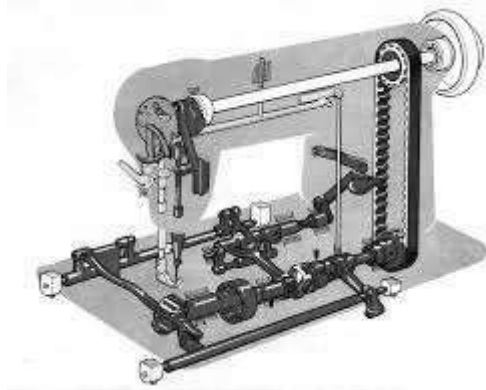
Мошинаи дарздӯзӣи ОЗЛМ ва сохти кинематикии он
