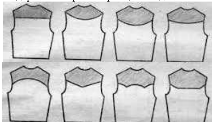
Навъҳои пайвасти камзӯлчаи ақиб ба тана
