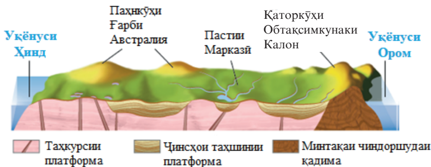
Сохти қири замин ва релйефи Австралия (30° а.ҷ.)
