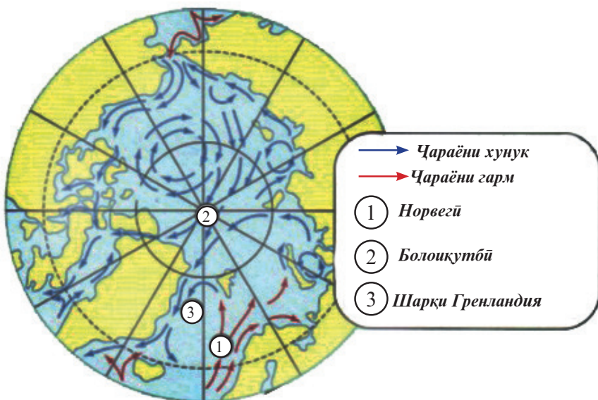
Нақшаи чараёнҳои уқёнуси Яхбастаи Шимолӣ
