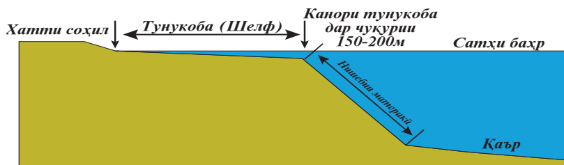
Буриши уқёнус дар назди соҳил
