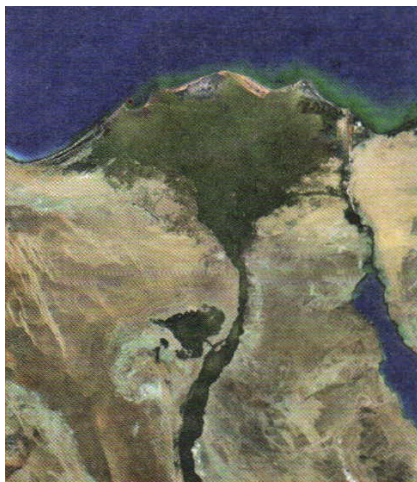
Делтаи дарёи Нил
