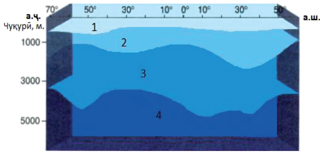
Анбӯҳҳои оби уқёнуси Атлантик (аз рӯйи буриши меридианӣ - аз 70° а.ч. то 60° а.ш.): 1 – сатҳӣ; 2 – мобайнӣ; 3 – чуқуроба; 4 – қаъри
