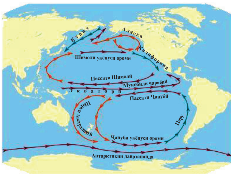
Чараёнҳои дар уқёнуси Ором
